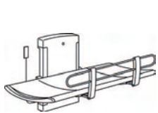
AQUACON CAMILLA DE ASEO CON MOTOR ELÉCTRICO
